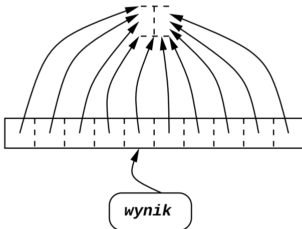
Rysunek 7.3. Sytuacja po drugim wierszu z Listingu 7.21 (przerywany symbol oznacza tu pustą listę)
