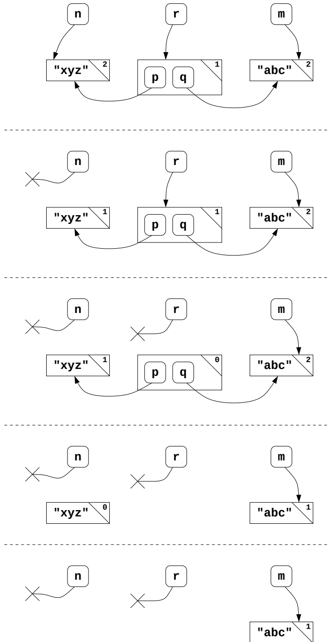
Rysunek 3.5. Sytuacja na sterze w Listingu 3.15; patrząc od góry: po linii 5; po linii 6; po linii 7 (etap I); po linii 7 (etap II); po linii 7 (etap III)
