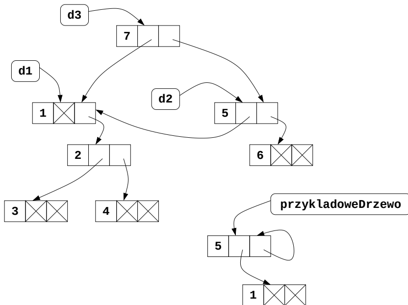
Rysunek 5.1. Reprezentacja w pamięci (nieco uproszczona) drzew przykładoweDrzewo, d1, d2, d3 z Listingu 5.11
