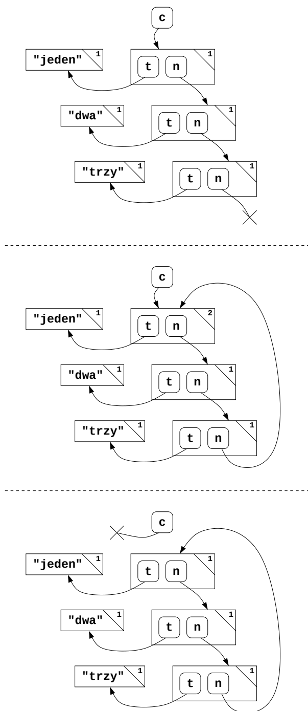
Rysunek 3.6. Sytuacja na stercie w Listingu 3.16, od góry: po linii 6; po linii 7; po linii 8
